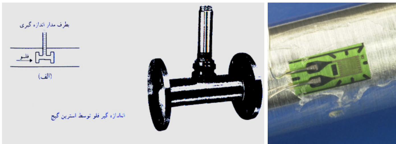
مدار استرین گیج بروی لوله
