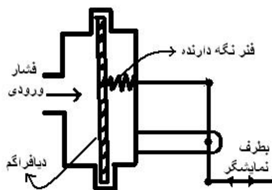
شکل ۲۲: اصول کار اندازه گیر فشار دیافراگمی
