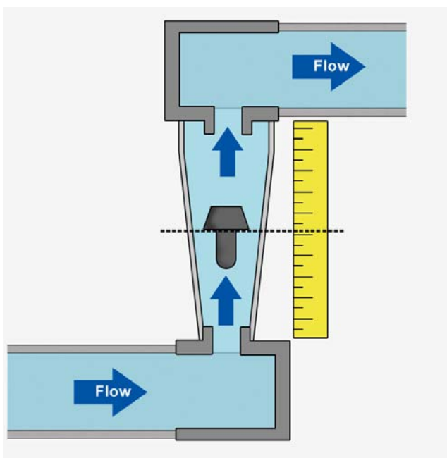
شکل ۲۹: روتامتر
