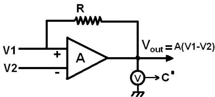
شکل ۱۷: تقویت کننده
