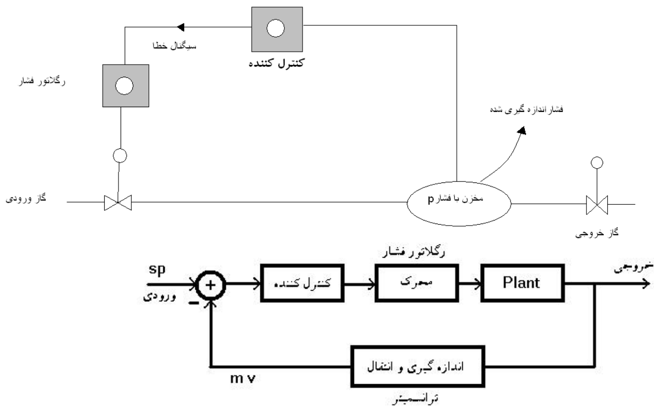
شکل ۲: سیستم کنترل فشار مخزن
