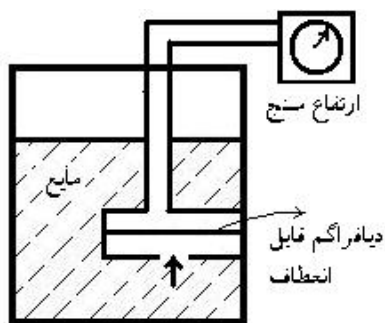
۵- اندازه گیری با استفاده از سطح سنج شیشه ای :
