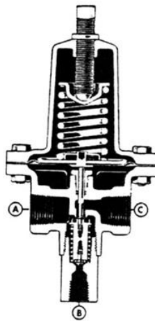
شکل ۲۴-۷ شیر حبسی که برای نگهداری شیر در آخرین موقعیت آن هنگام بروز خطا در هوای تغذیه استفاده می‌شود.
