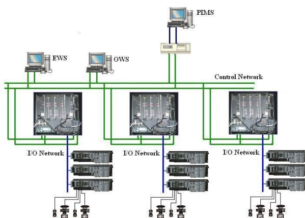
شکل ۹-۵ ساختار کنترلی غیرمتمرکز (Distributed Control System)
