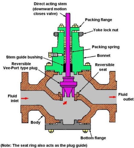
شکل ۷-۴- شیر تک‌ورودی غیرمتعادل معکوس‌پذیر پلاگ‌دار
