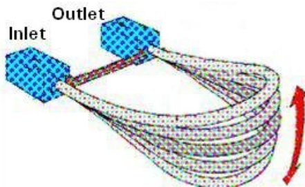
شکل ۵-۱۴ فلومتر کرولیس
