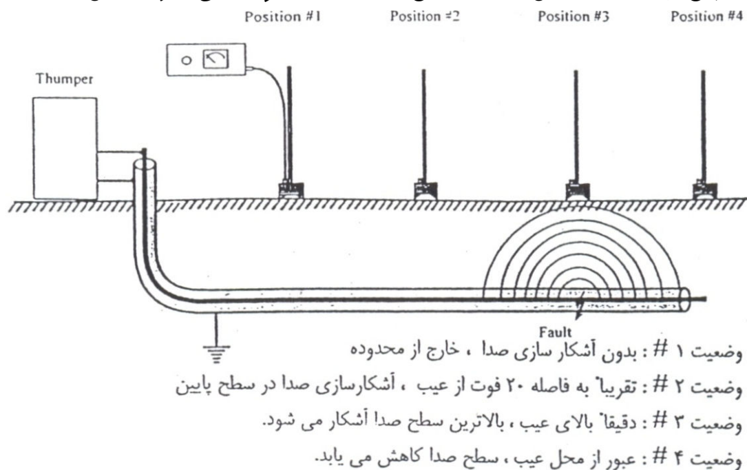
شکل ۱۲: آشکار سازی موج ضربه آکوستیک
