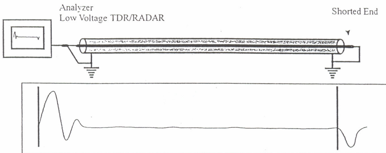
شکل ۳۵ استفاده از آنالایزر برای اندازه گیری طول کابلی که انتهای آن اتصال کوتاه شده است.
