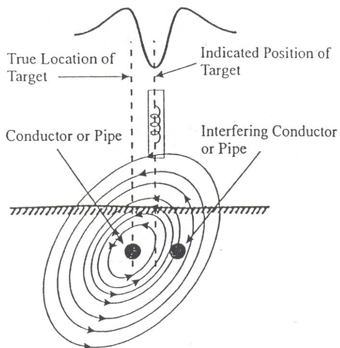
شکل ۲۸: اختلاف ناشی از تداخل کابل به غیر از کابل تحت آزمایش
