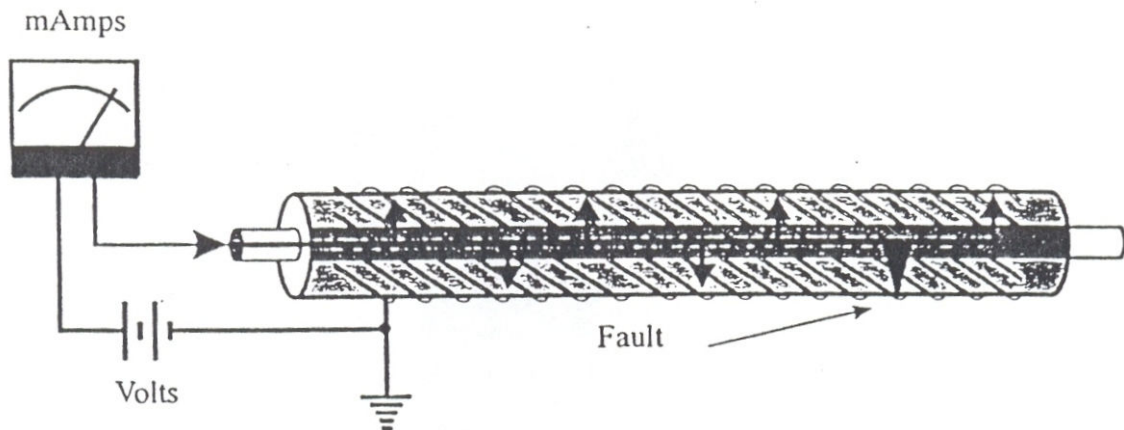
شکل ۳۱: کابل معیوب
