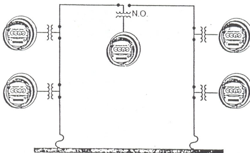
شکل ۴۶: سیستم حلقوی URD
