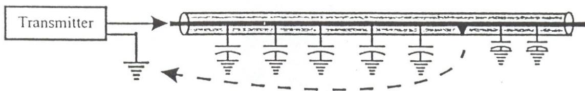
شکل ۲۰: Hook up بدون میله زدن در سر انتهایی کابل تحت آزمایش
