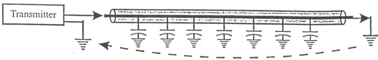
شکل ۱۹: Hookup نشان دهنده میله زمین در سر انتهایی کابل تحت آزمایش
