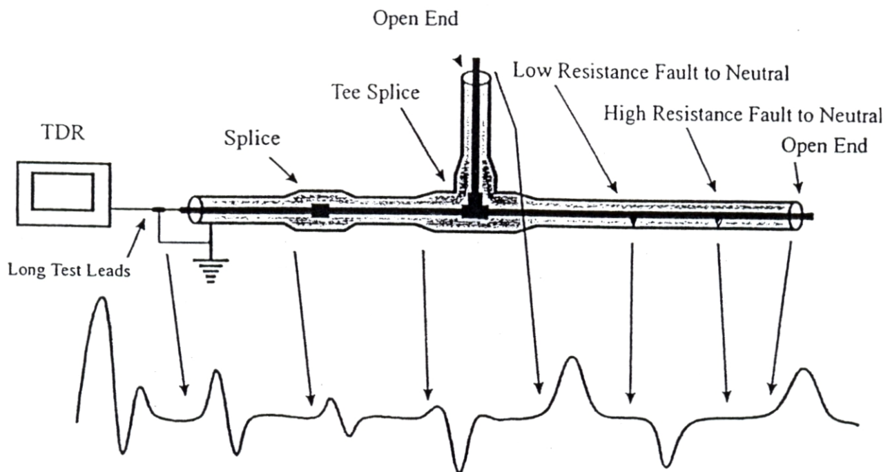
شکل ۸: کاربرد TDR روی کابل قدرت
