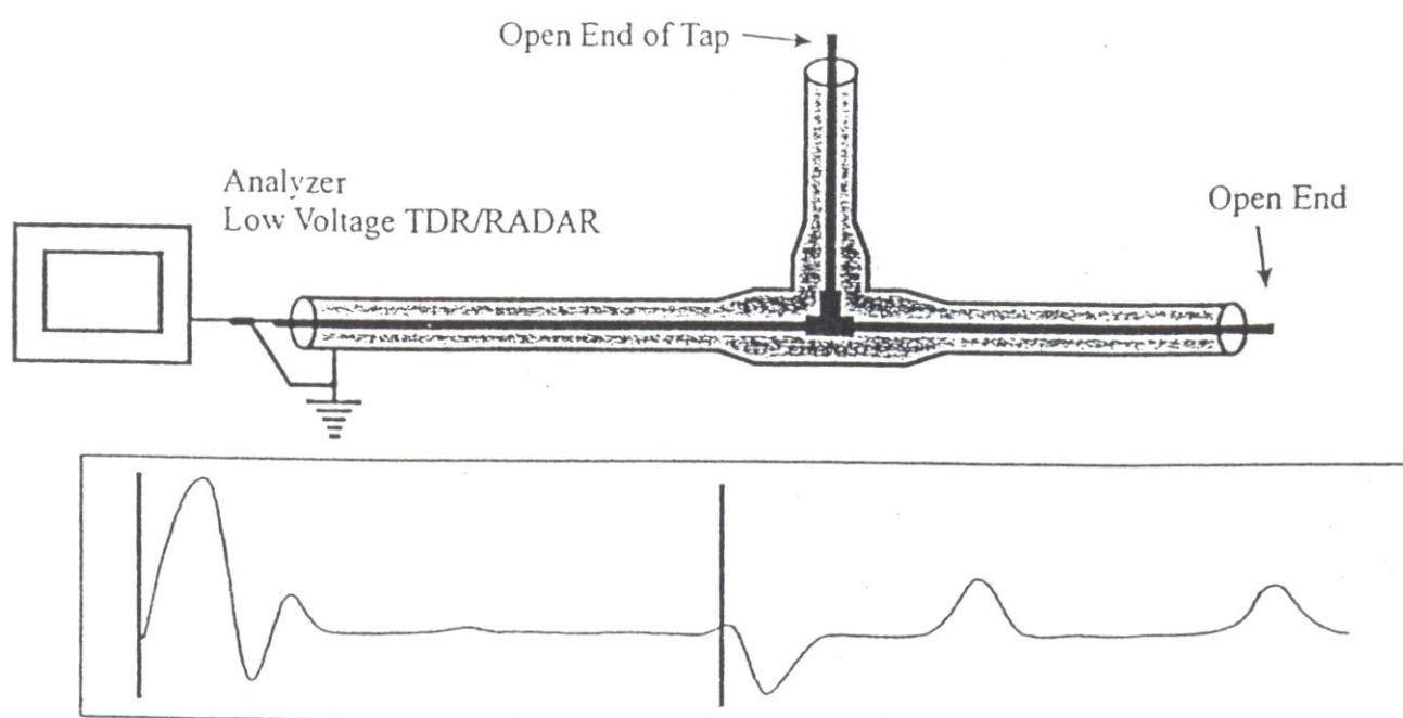
شکل ۳۹: کاربرد آنالایزر برای تعیین جای تقریبی یک تپ Y
