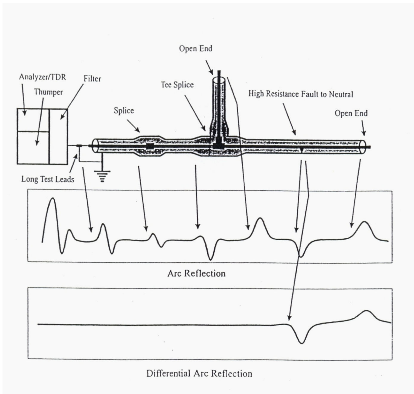
شکل ۹: روشهای انعکاس قوسی و انعکاس تفاضلی رادار ولتاژ قوی
