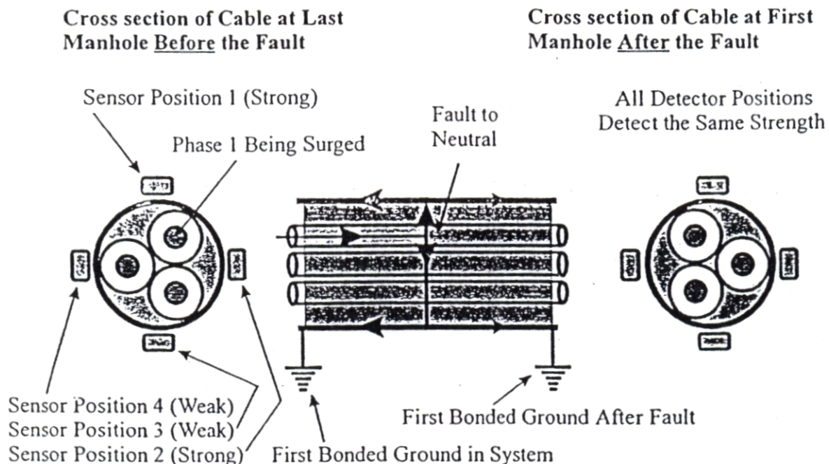
شکل ۷: آشکارسازی الکترومغناطیسی عیوب در کابل قدرت سه فاز
