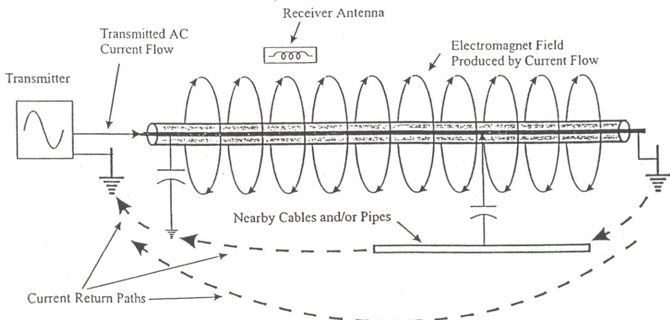
شکل ۱۶: نحوه کار محل عیب یاب کابل
