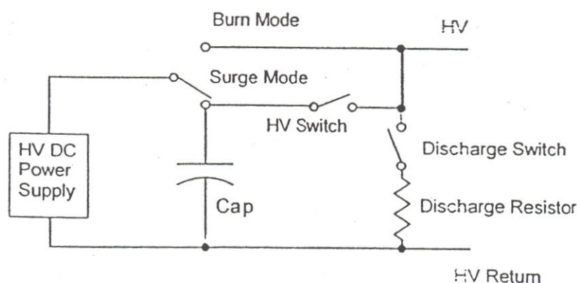
شکل ۴۲: نمودار بلوکی ژنراتور موج ضربه
