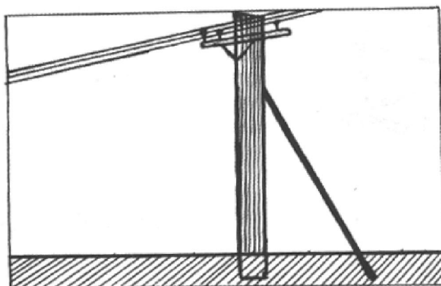
شکل ۲۶- مهار تودلی
