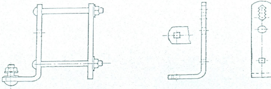
شکل ۱ - دستک نصب نوع «بی»
