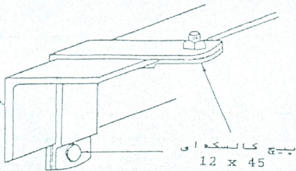
کنسول فولادی 100 x 100 x 10
