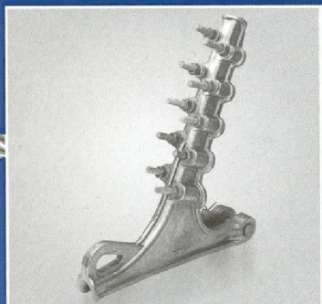
کلمپ انتهایی ۱۲۰-۱۹۵ کپی داخل (دیکست) >> مورد تایید شرکت توزیع برق شیراز
