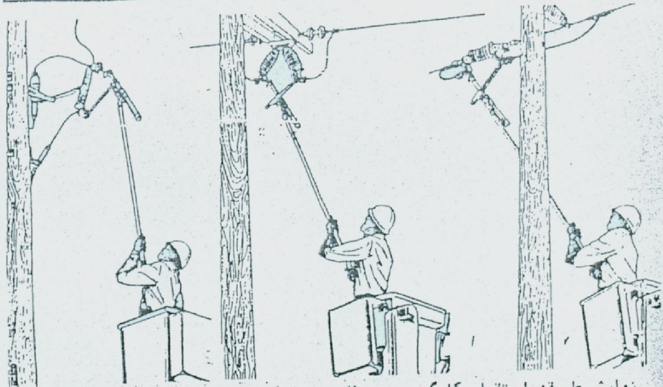
نمایش طریقه استقرار کارگر درون بالابر برای کاربرد لودبوستر جهت سیستم توزیع هوایی
