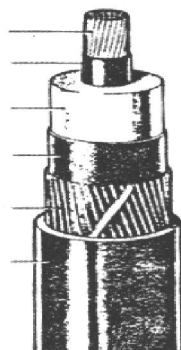
شکل ۳۰- ب- نمونه ای از کابل pex تک هسته 12-170\text{ kV}
