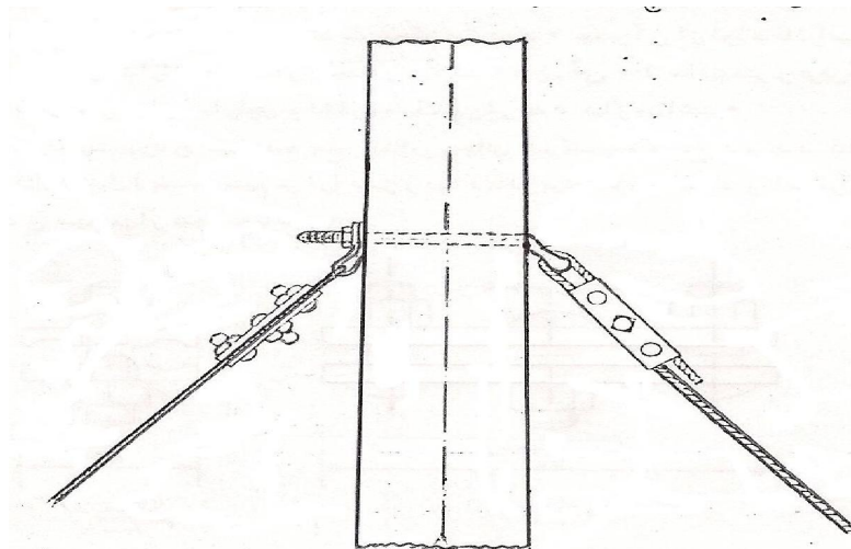
پیچ زاویه دار و گوشواره زاویه دار
