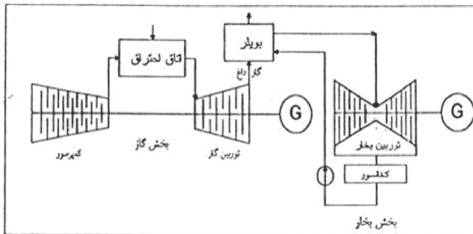
شکل زیر شمای عمومی نیروگاههای سیکل ترکیبی را نشان می دهد :
