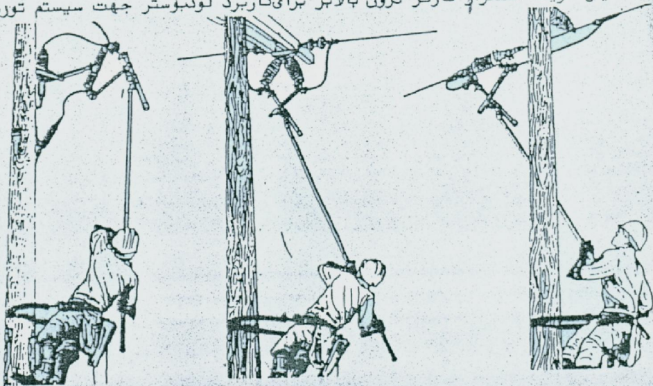
نمایش طریقه استقرار کارگر بر روی پایه جهت استفاده از لود بوستر برای سیستم توزیع هوایی
