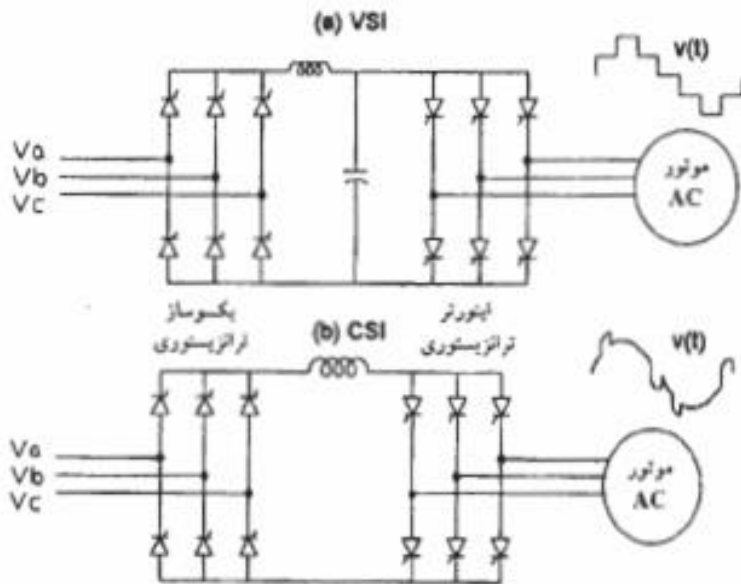
شکل ۶-۱۳: محرکه‌های با قدرت بالا
