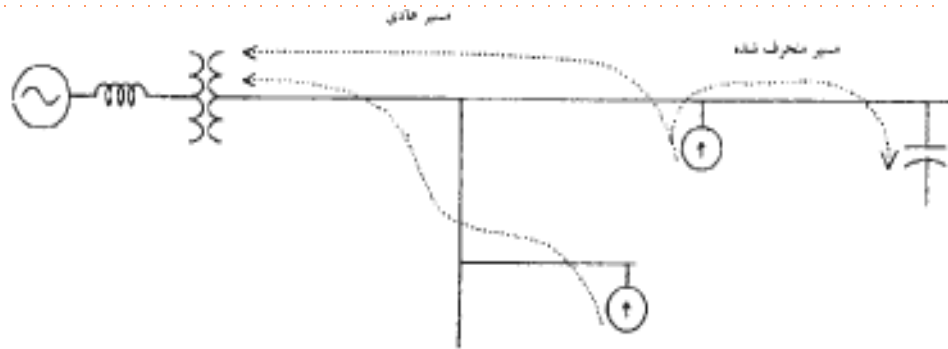
شکل ۲۸-۶: خازنهای تصحیح ضریب قدرت قادر به تغییر مسیر یکی از مؤلفه‌های هارمونیک جریان هستند
