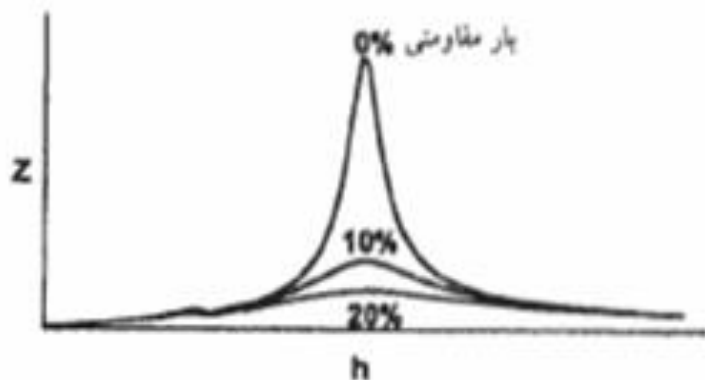
شکل ۴-۲۶: تأثیر بارهای مقاومتی روی پدیده تشدید موازی
