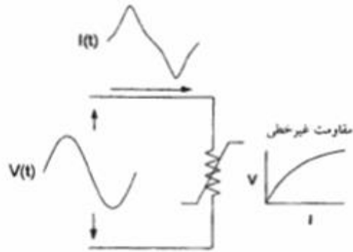
شکل ۱-۲: اعوجاج جریان که به علت یک مقاومت غیرخطی ایجاد شده است
