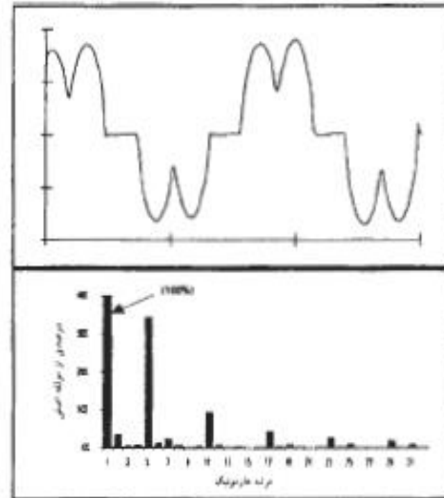
شکل ۹-۶: طیف هارمونیکی یک محرکه AC از نوع CSI
