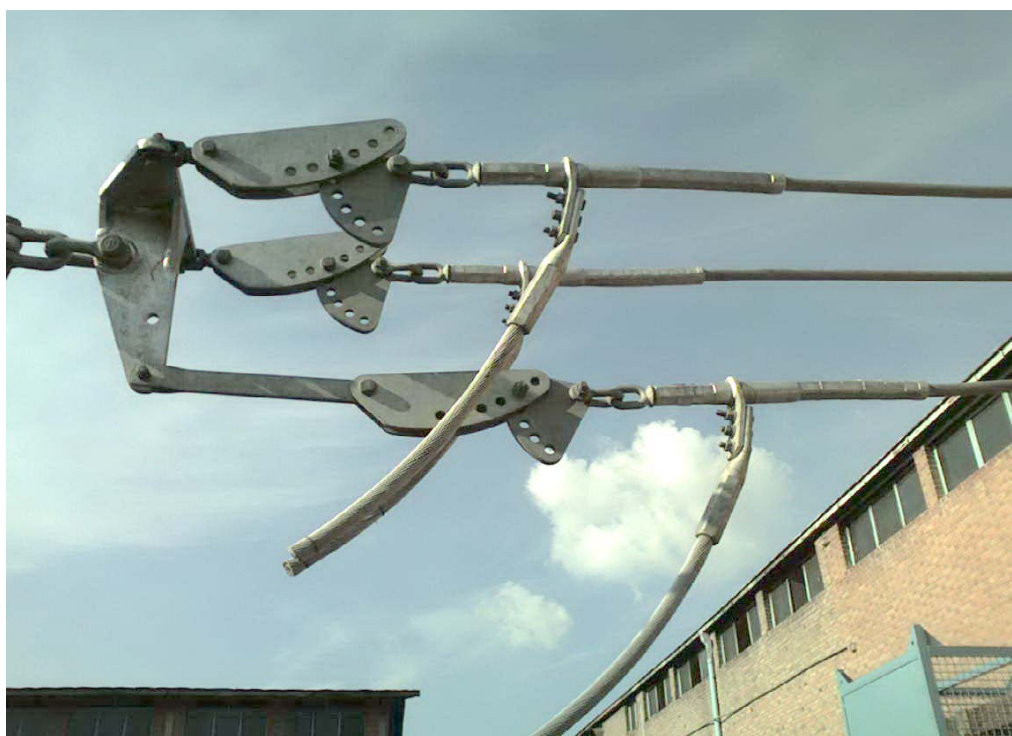
شکل ۳۹) استفاده از , Shackle , Extension Link , Socket Clevis , Yoke Plate
