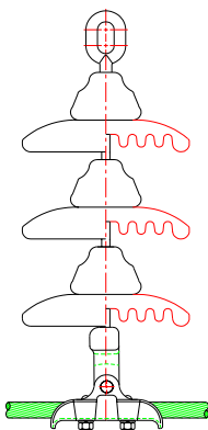
شکل ۳۳) فاصله خزشی مقره
