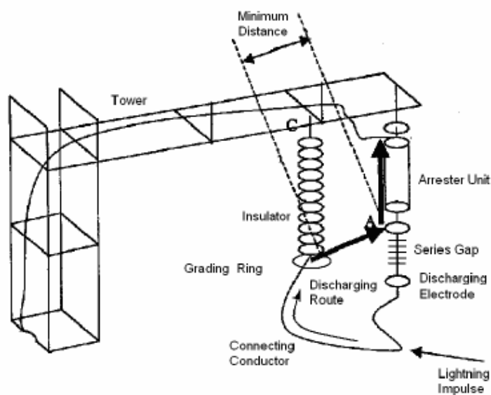
شکل ۴۴) مکانیزم استفاده از برقگیر خط بر روی دکل
