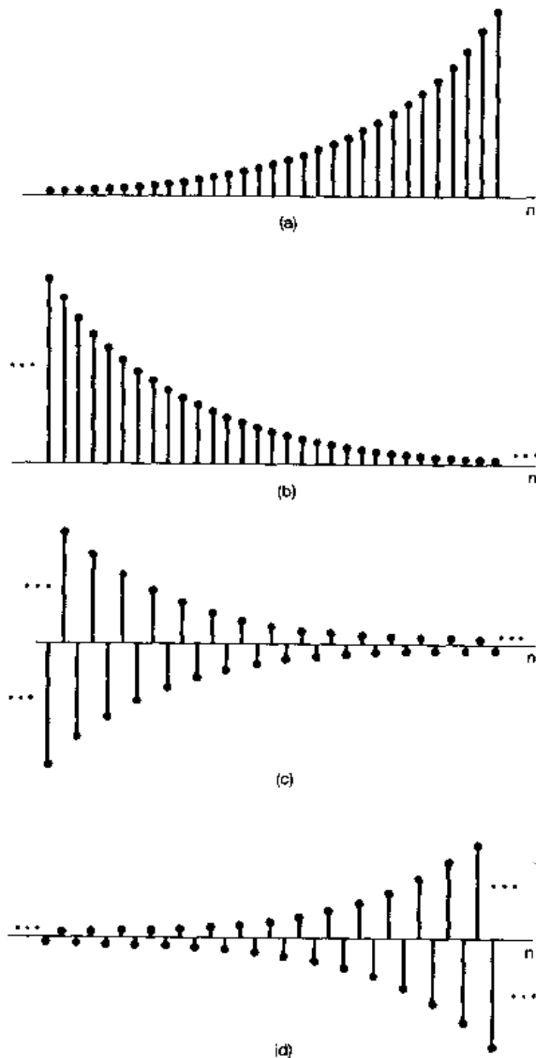
Figure 1.24 The real exponential signal x[n] = Ca^n : (a) \alpha > 1 ; (b) 0 < \alpha < 1 ; (c) -1 < \alpha < 0 ; (d) \alpha < -1
