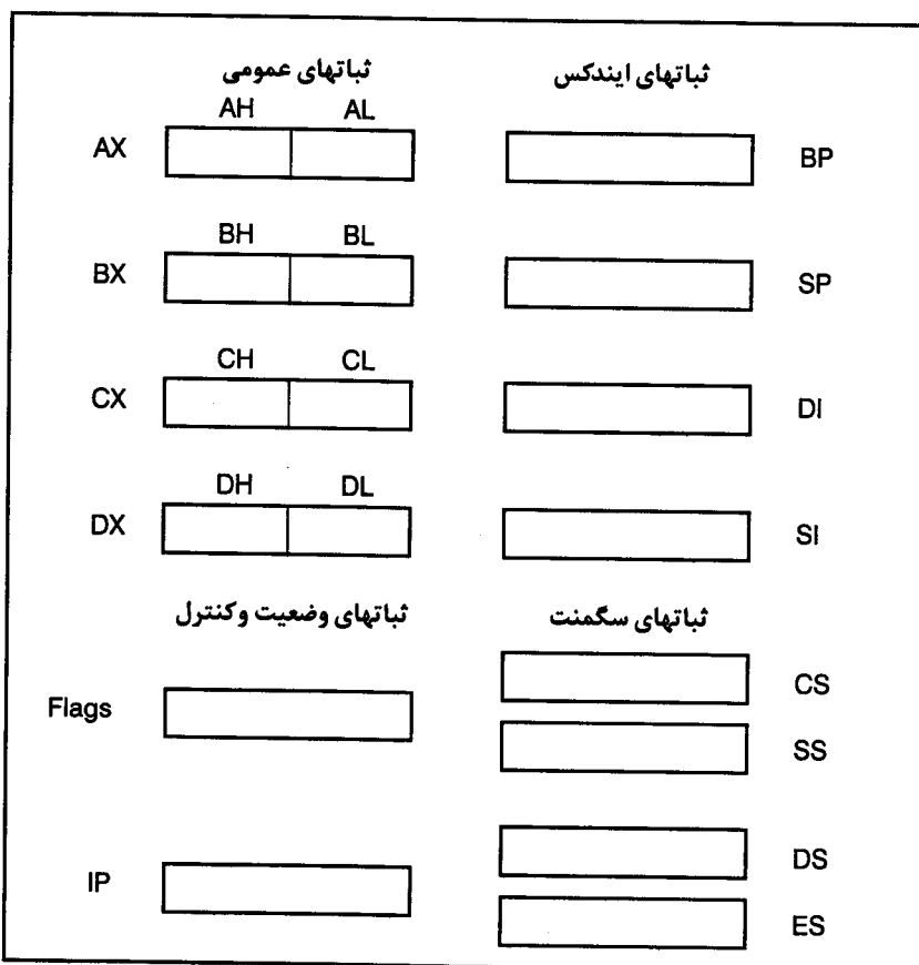
شکل ۲-۱۲ ثباتهای ۱۶ بیتی.
