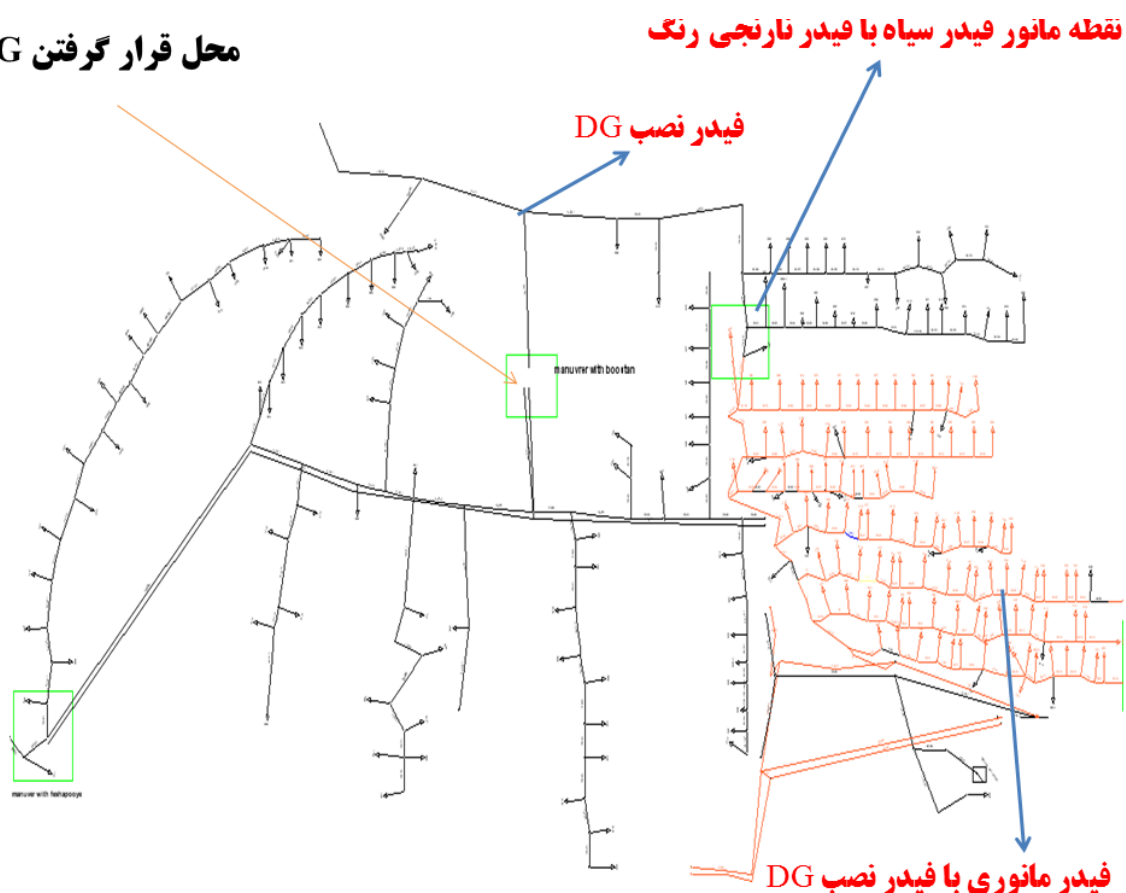
شکل (۵-۶): شبیه سازی فیدر نصب DG و فیدر مانوری با آن
