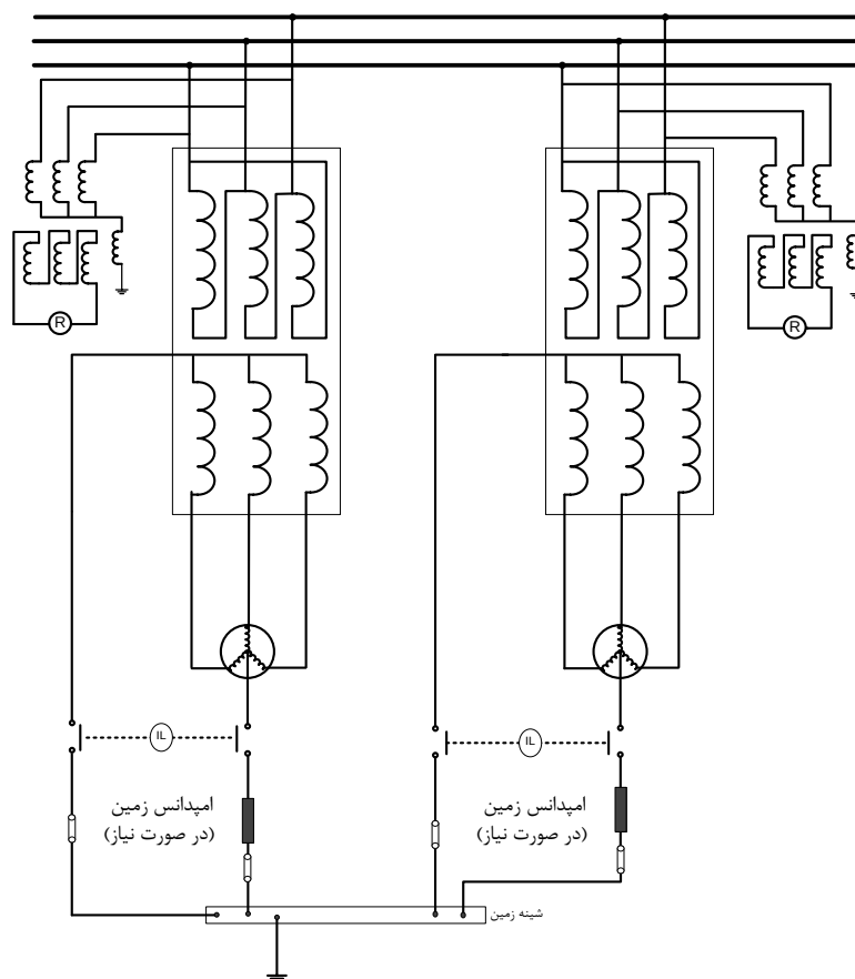
شکل (۷-۸): دو یا چند منبع تولید پراکنده به صورت موازی و جدا از شبکه دارای ترانسفورماتور مثلث-ستاره زمین شده
