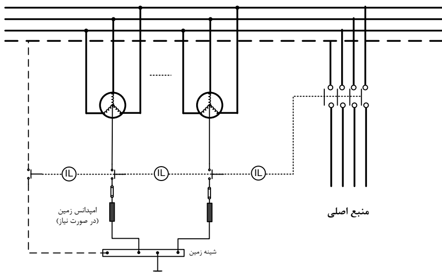
شکل (۸-۳): اتصال زمین دو یا چند مولد با قابلیت کار موازی با شبکه
