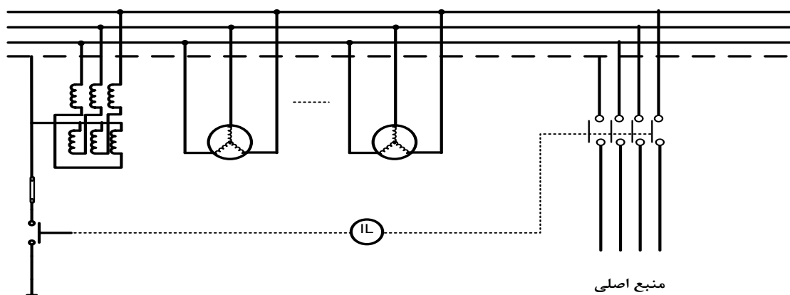
شکل (۸-۴): زمین کردن منابع تولید پراکنده که قابلیت کار موازی با شبکه را دارند به همراه ترانسفورماتور زمین
