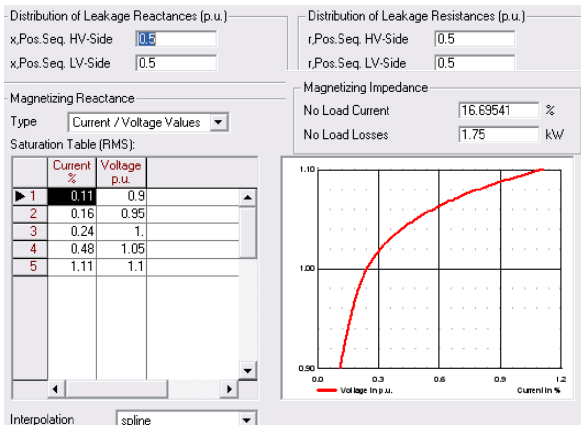
شکل (۵-۵): منحنی اشباع و راکتانس پراکندگی ترانسفورماتور
