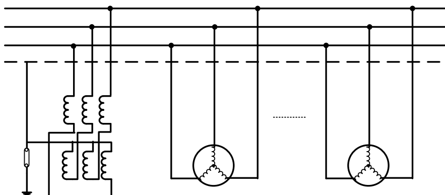
شکل (۸-۲): یک یا چند مولد موازی با ترانسفورماتور اتصال زمین
