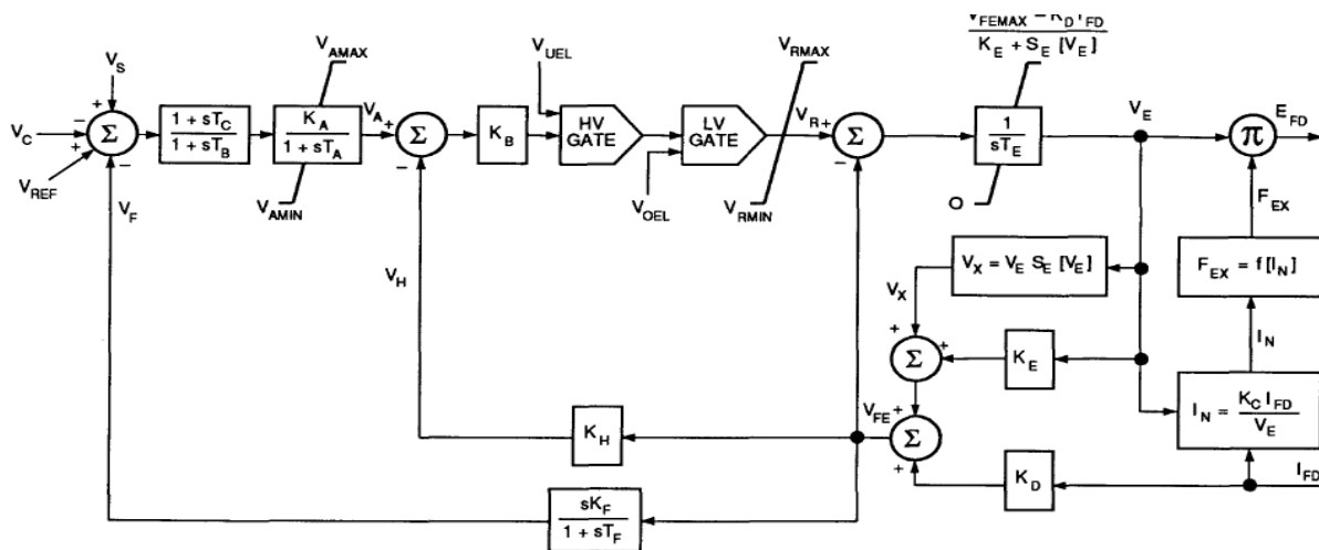
شکل (۵-۱۰): مدل سیستم تحریک ACA2
